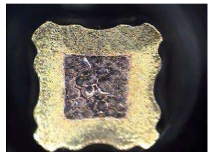
Beispiel Sondercrimp 4kant Example special square crimp
